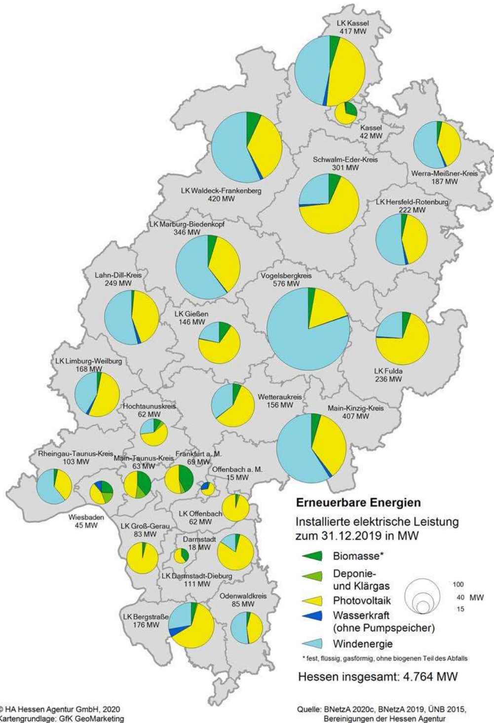
Abbildung 38: Installierte elektrische Leistung von nach EEG geförderten erneuerbaren Energieanlagen am 31.12.2019 in den hessischen Landkreisen und kreisfreien Städten nach Energieträgern (in MW)
